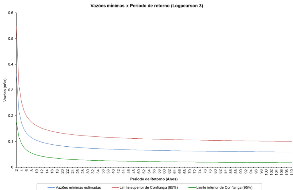
Figura 3-26 - Gráfico da vazão mínima associada a cada período de retorno estimado pela distribuição de Log Pearson 3 para a estação Itaguaçu – Jusante – rio Santa Joana.
