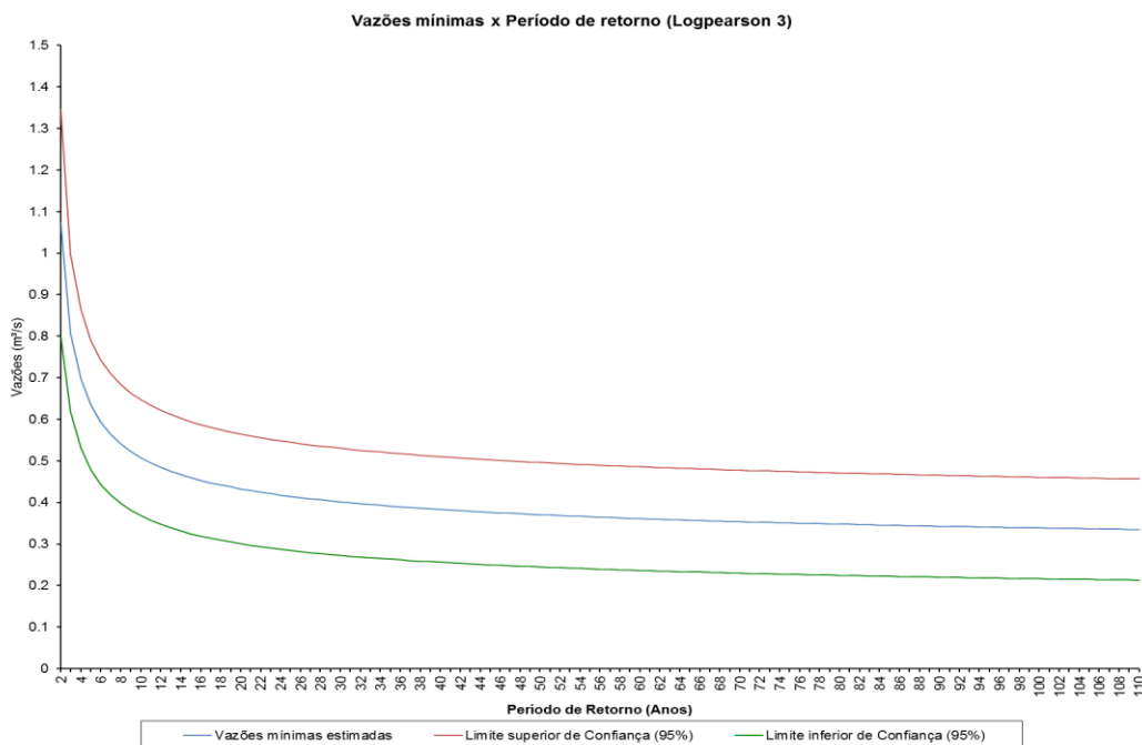
Figura 3-27 - Gráfico da vazão mínima associada a cada período de retorno estimado pela distribuição Log Pearson 3 para a estação Jusante Córrego da Piaba - rio Santa Joana.
