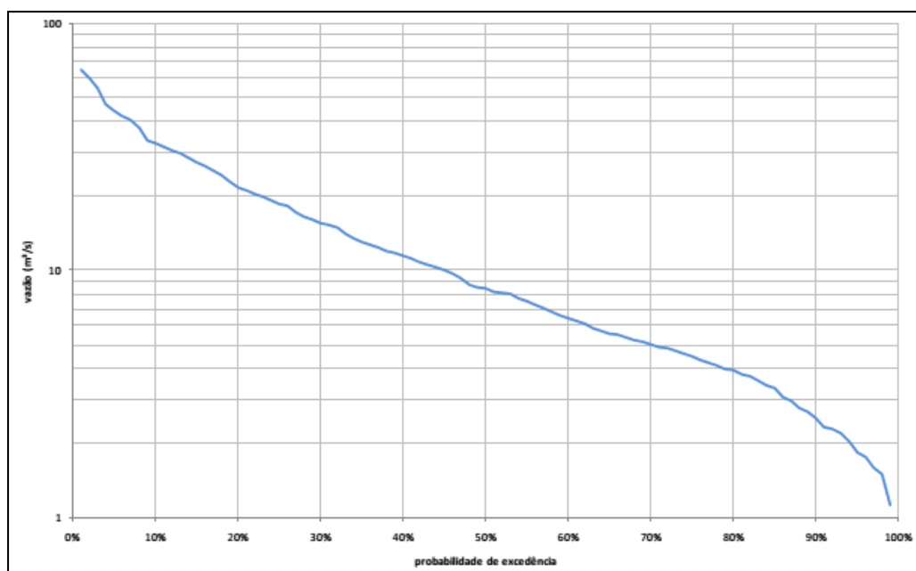
Figura 3.11: Curva de Permanência das vazões médias diárias - Rio Pancas.
